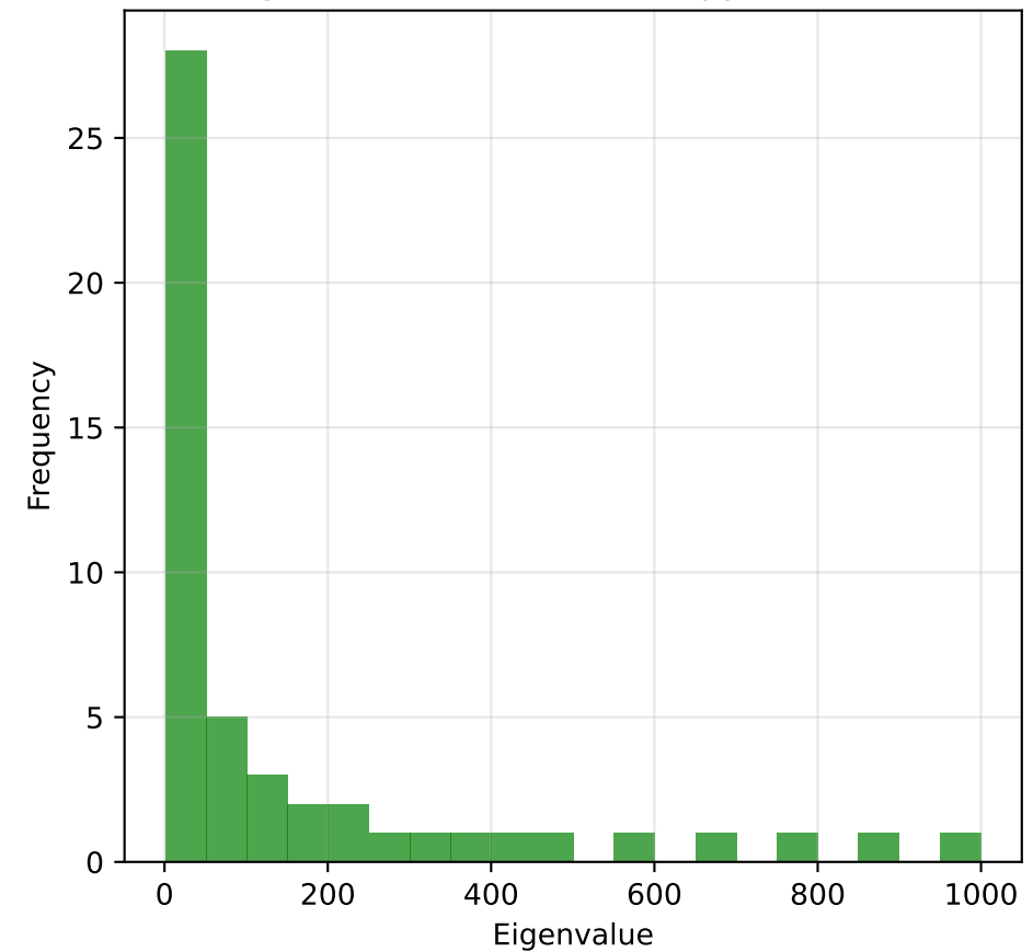
Eigenvalue Distribution (kappa = 1000)
