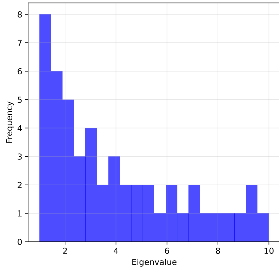
Eigenvalue Distribution (kappa = 10)
