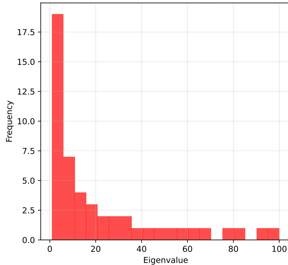
Eigenvalue Distribution (kappa = 100)
